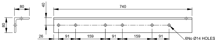
TPL-B-1 - EA 80x80x8 Scale 1:10
